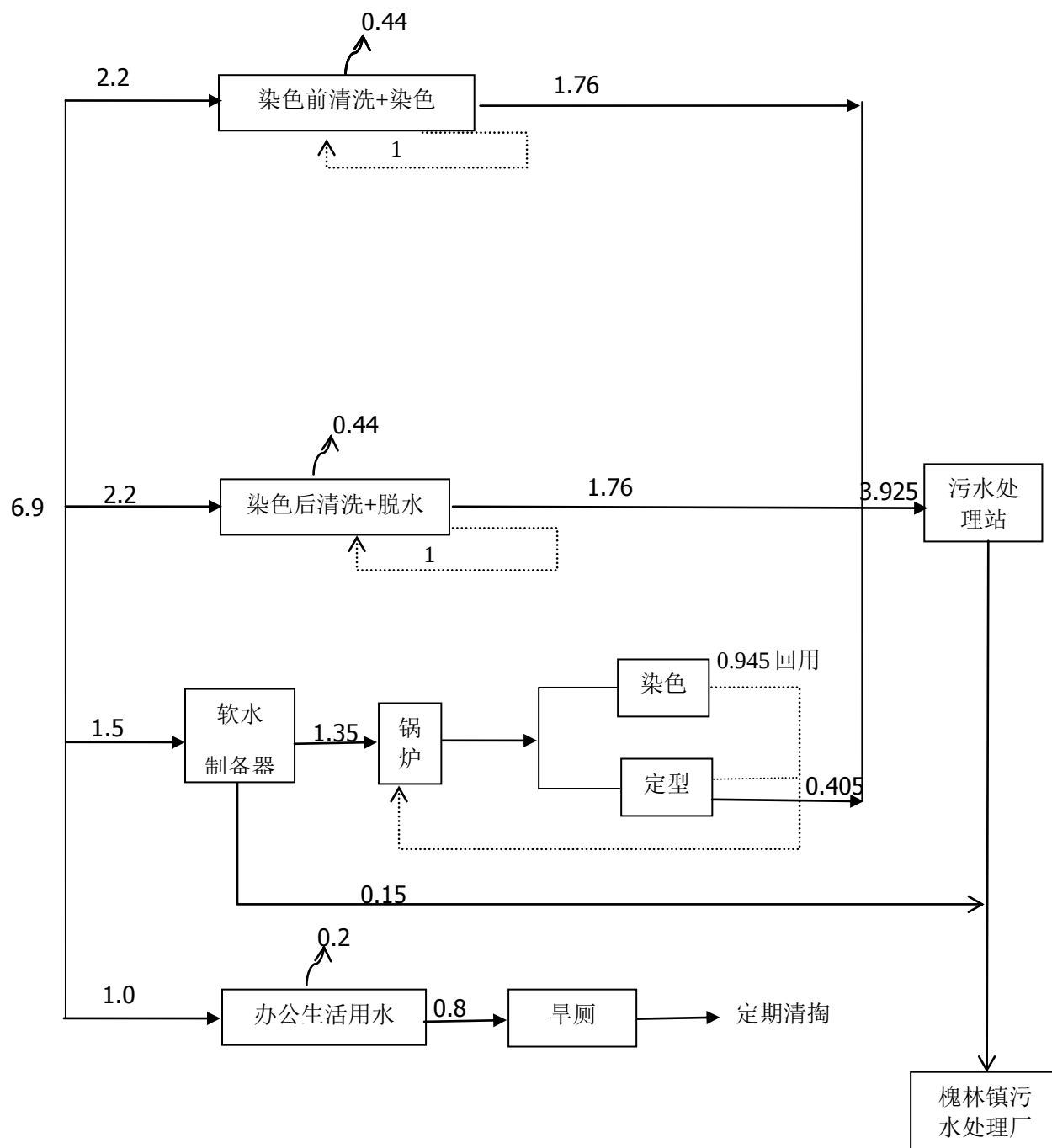
图 3.5-1 项目水平衡图
