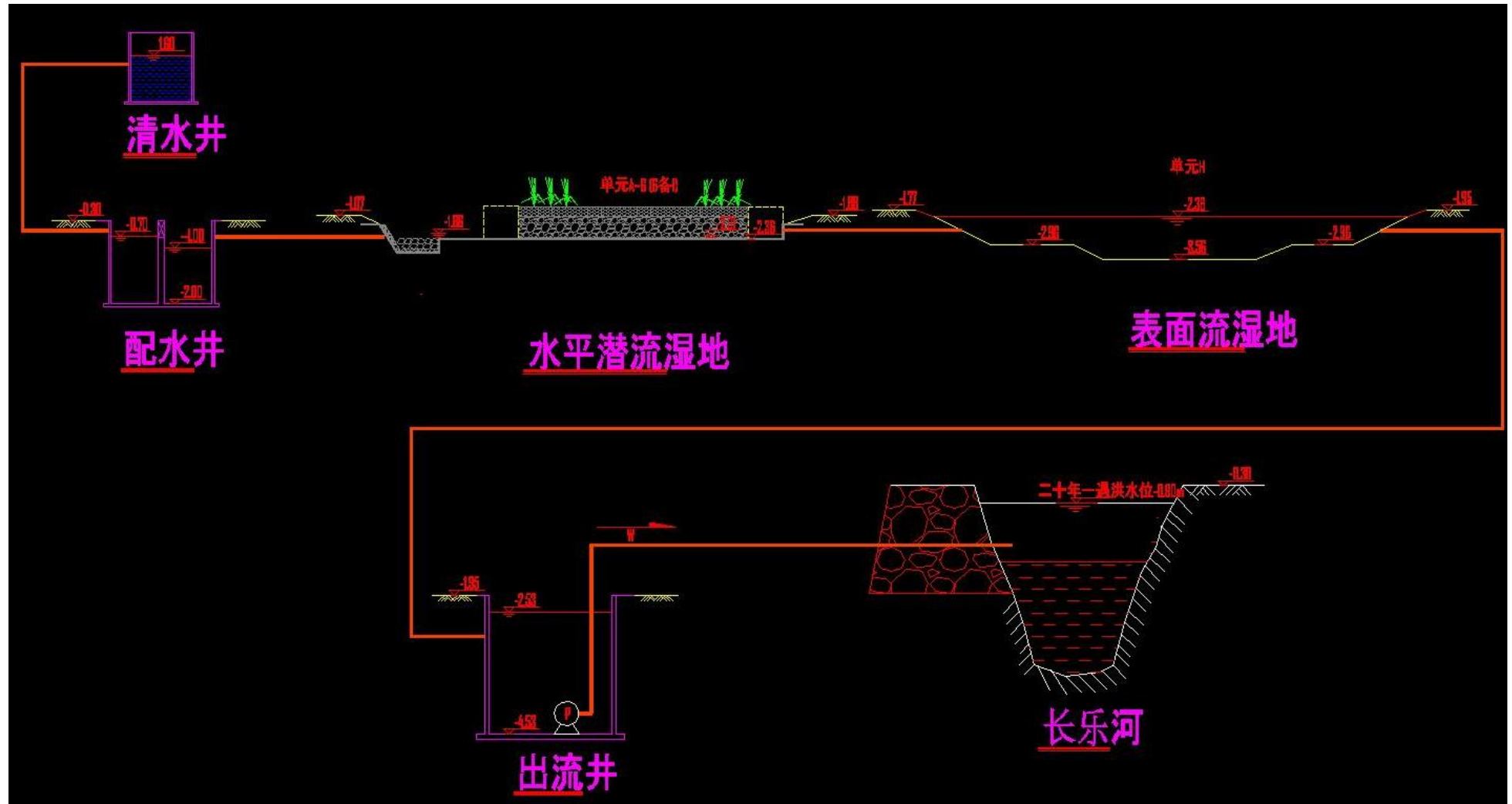
附图 4 项目工艺高程图
