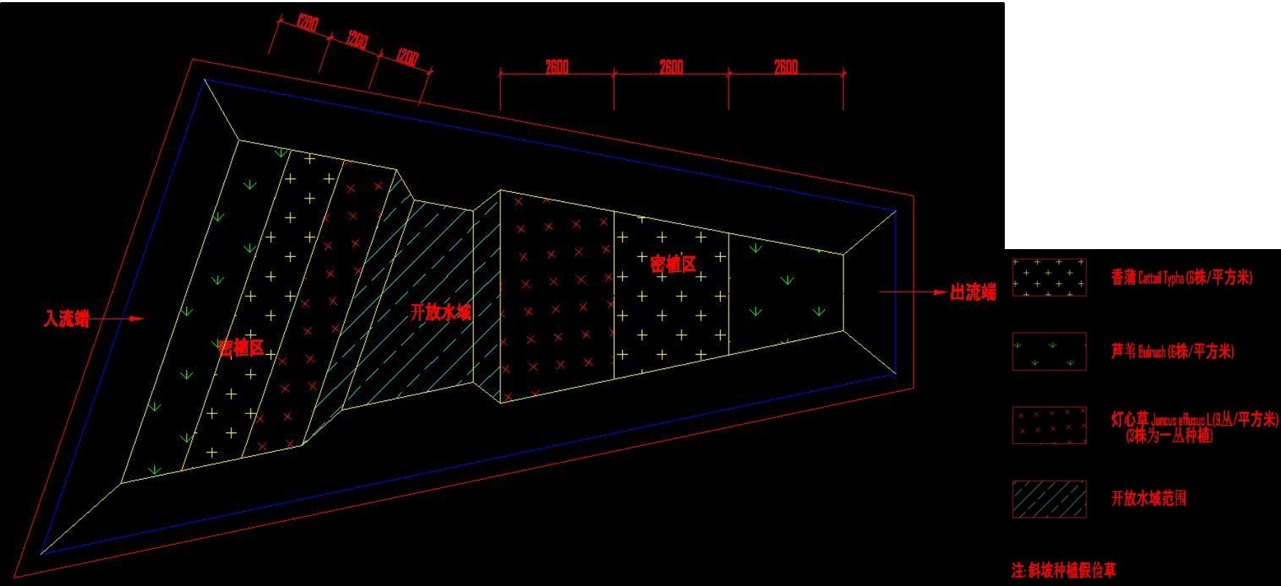
单元 F 平面配置图
