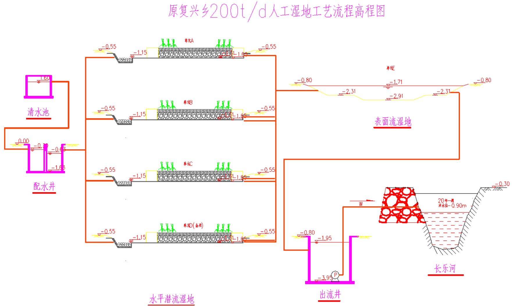
附图 4 项目工艺高程图
