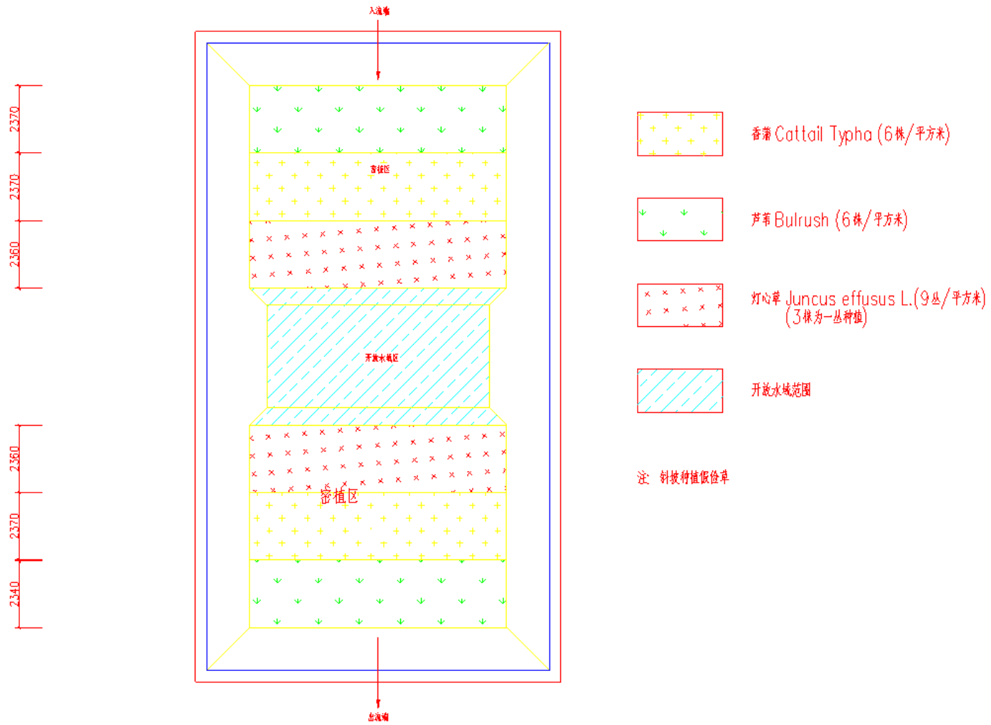
单元E 栽植配置图
