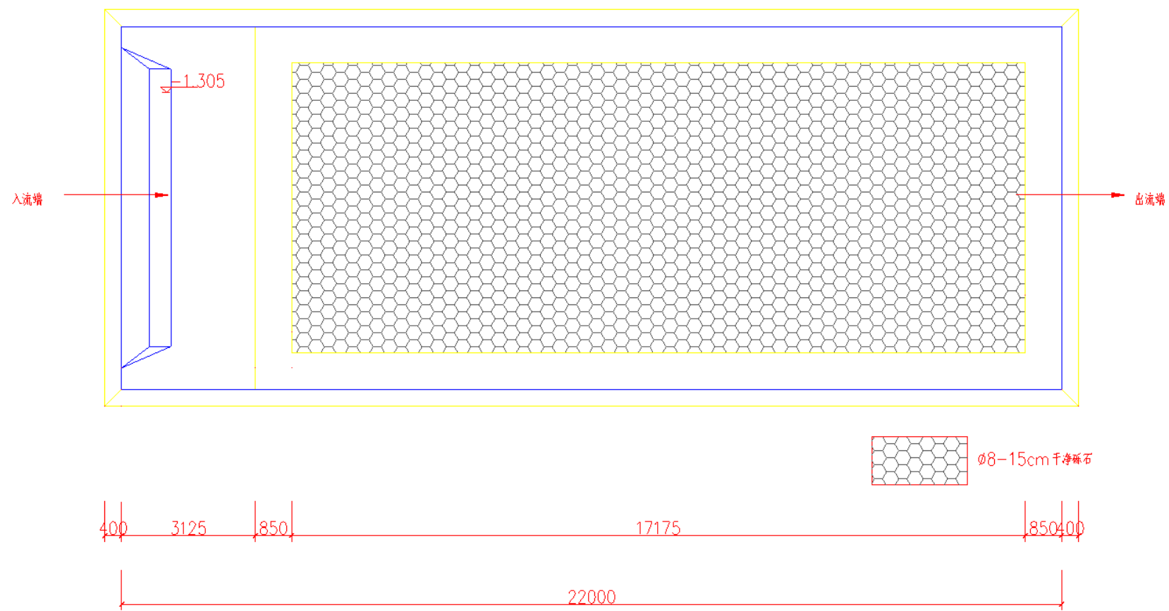
附图 5 湿地各单元配置图
