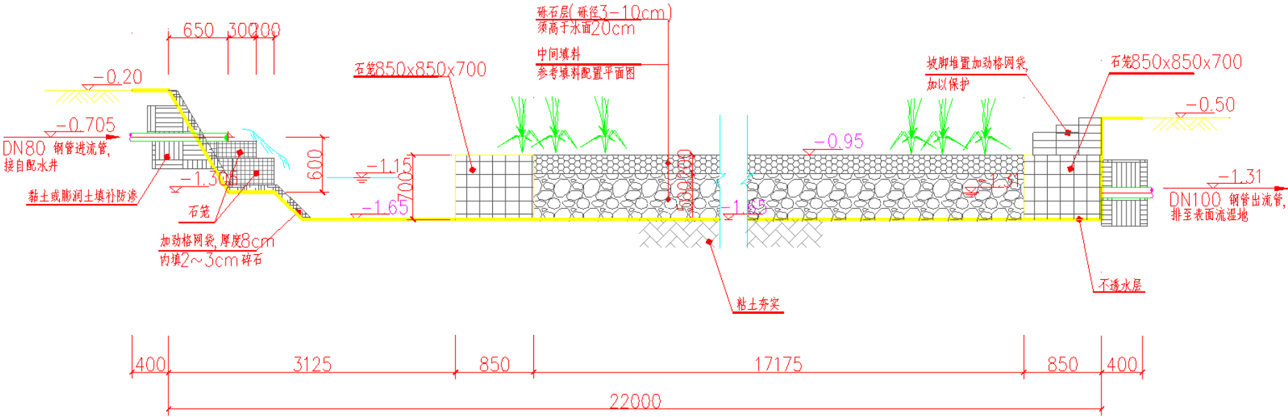
单元A |—| 剖面图
